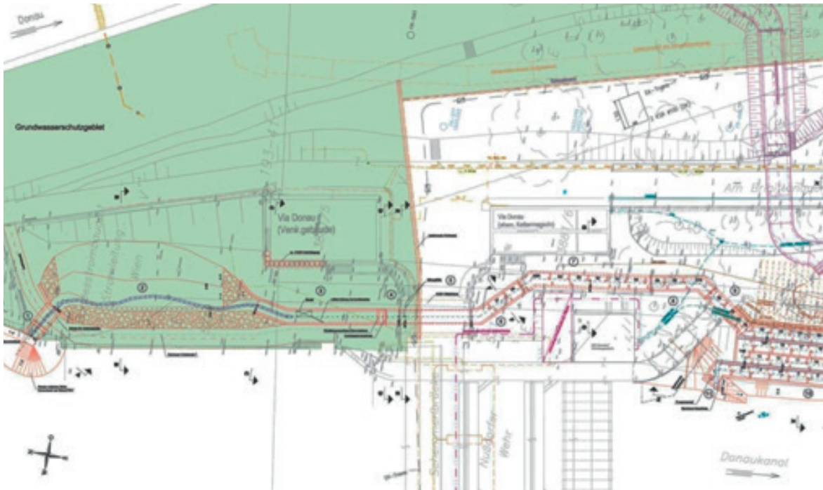
Einreichungsplan der Fischaufstiegshilfe Nußdorf
